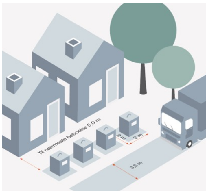
Figur 1B: Illustration af krav til placering af delvist nedgravede affaldsløsninger
