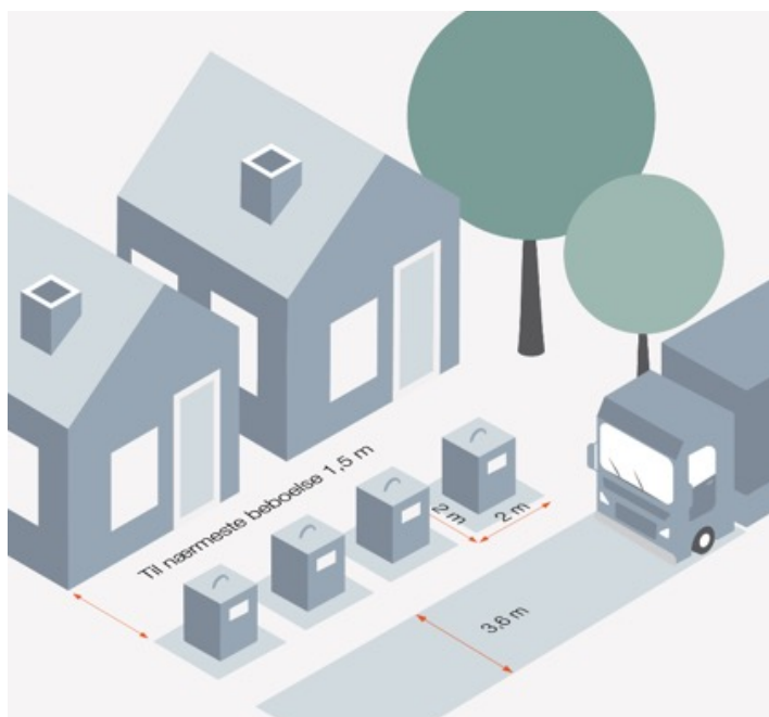
Figur 1A: Illustration af krav til placering af fuldt nedgravede beholdere og kuber
